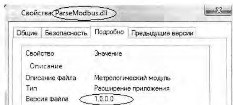
Рисунок 7 - Идентификационные данные ПО «Пирамида 2000», модуль обработки значений физических величин, передаваемых по протоколу Modbus
