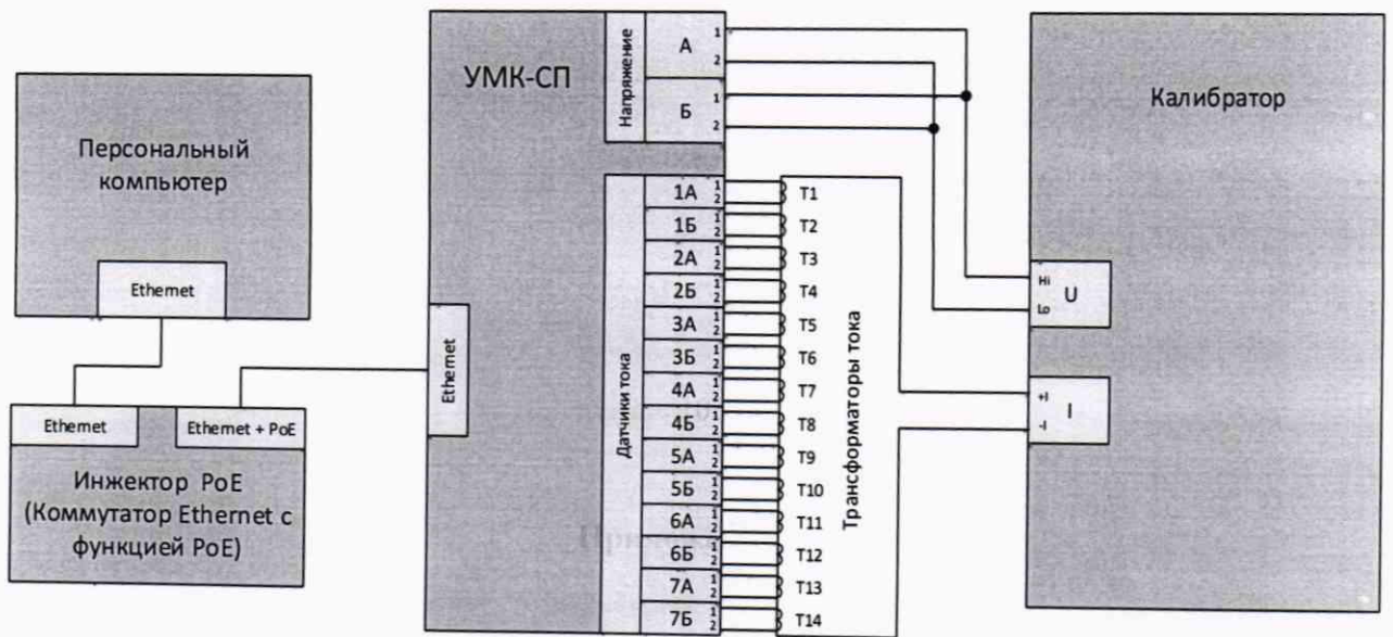
Рисунок А.1 – Схема подключения для проверки метрологических характеристик
