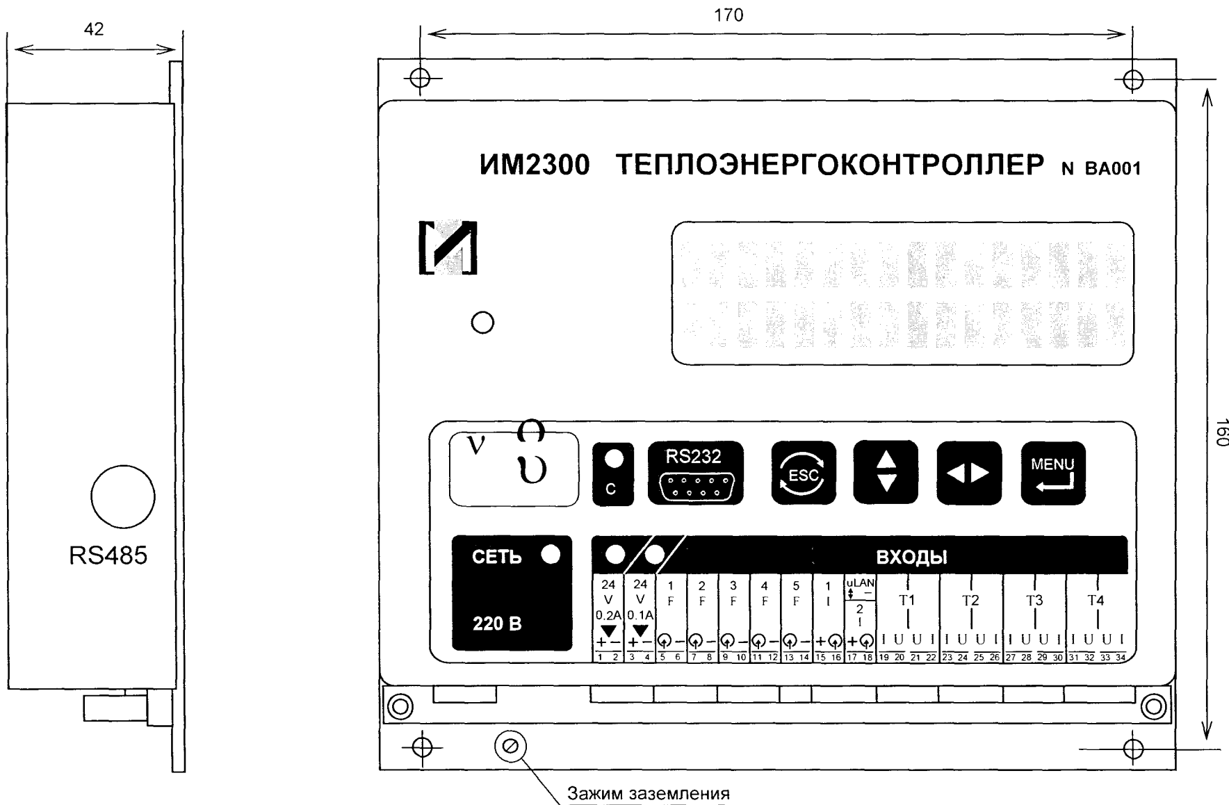
Рисунок 2.2 Органы управления, индикации и коммутации прибора ИМ2300Н1-5F
