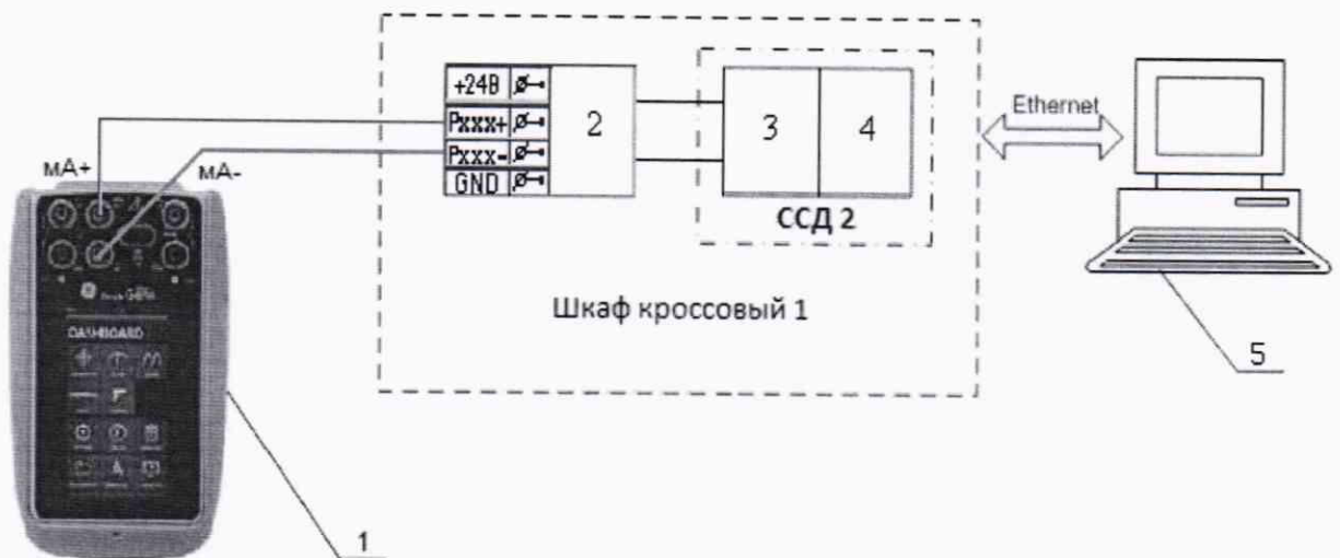
Рисунок 21а - Функциональная схема поверки ИК силы постоянного тока (ССД-1)
