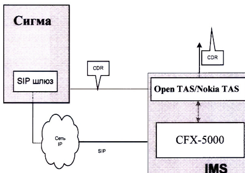
Рисунок 1- Схема поверки
