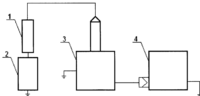
Рис. 2 – Схема измерений при определении погрешности измерения силы постоянного и переменного тока
