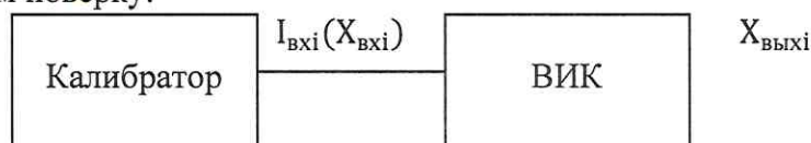
Рисунок 2 - Схема подключения при определении МХ ВИК преобразования сигналов постоянного тока в диапазоне от 4 до 20 мА
