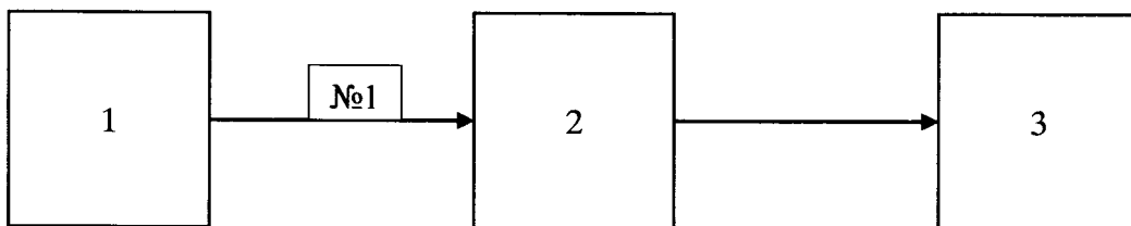
Рисунок А.2 – Функциональная схема для определения погрешности эклектической части ИК избыточного давления (для каналов А-У)
