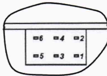
Рисунок В.2 – Схема расположения контактов разъема на боковой стороне корпуса счетчика вариант 12 серии 05, 06, 07
