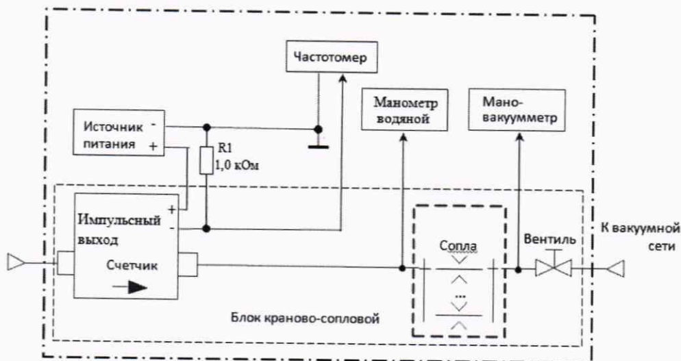
Рисунок А.3 – Схема проверки импульсного выхода на аналогичных установках поверочных
