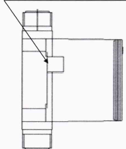
Рисунок 2 – Схема пломбировки от несанкционированного доступа, обозначение места нанесения знака поверки счетчиков СГ-1 вариант 12 серии 01 и 02
