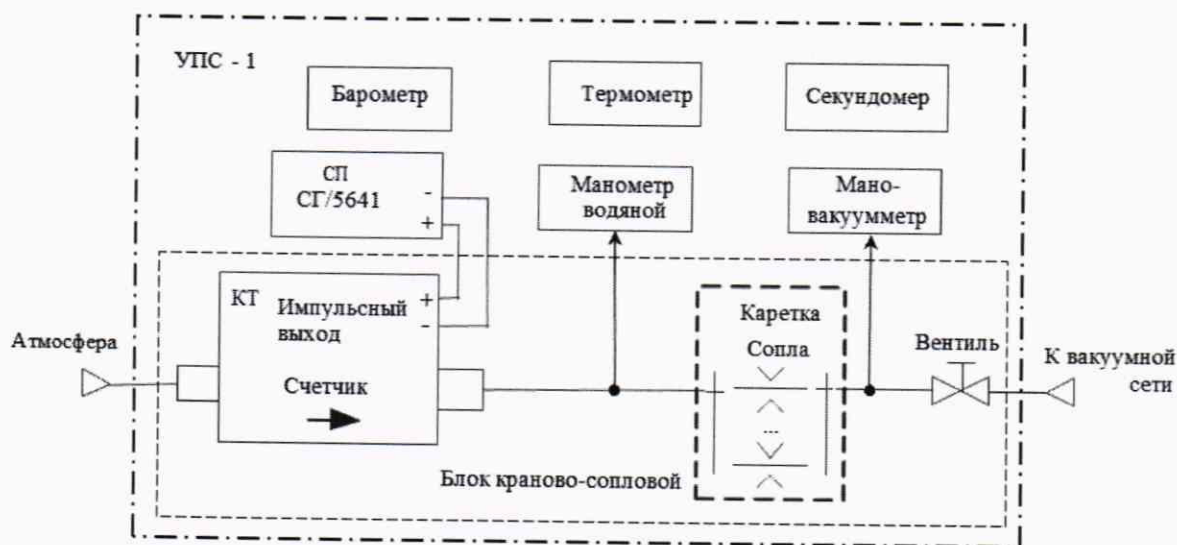
Рисунок А.2 – Схема поверки импульсного выхода на установке поверочной УПС-1
