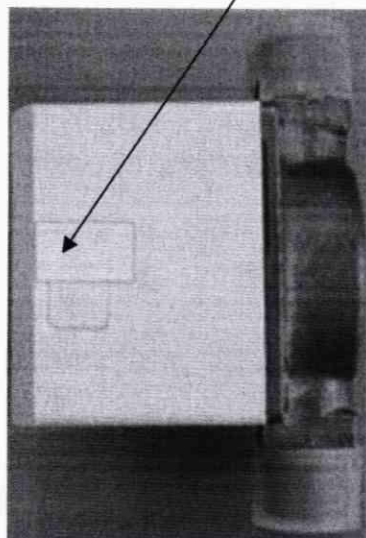
Рисунок 3 – Схема пломбировки от несанкционированного доступа, обозначение места нанесения знака поверки счетчиков СГ-1 вариант 12 серии 05, 06, 07
