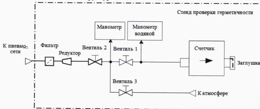
Рисунок А.1 – Схема проверки герметичности
