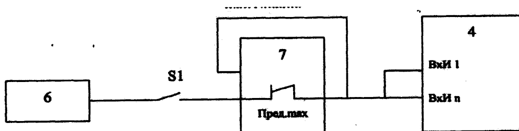
Рисунок А.3.1 – Схема определения погрешности при измерениях количества импульсов
