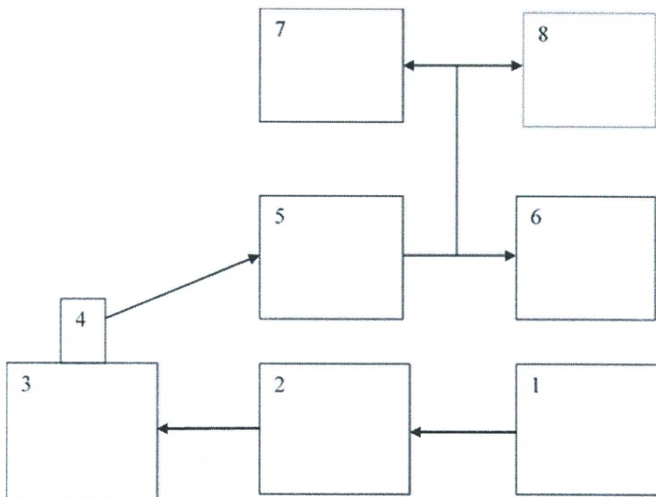
Рисунок 2 - Блок-схема виброустановки при определении коэффициента гармоник виброускорения.
