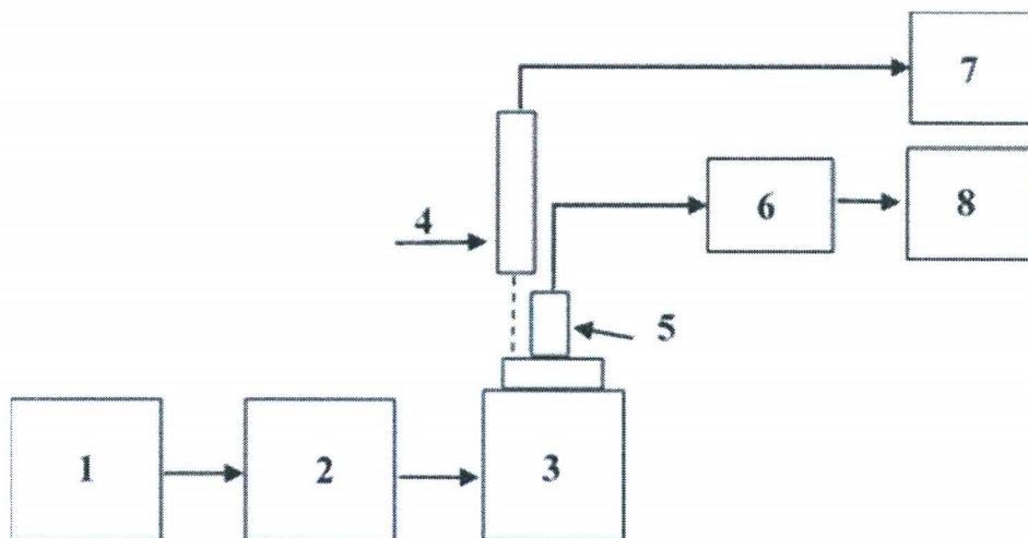
Рисунок 1 - Блок-схема виброустановки
