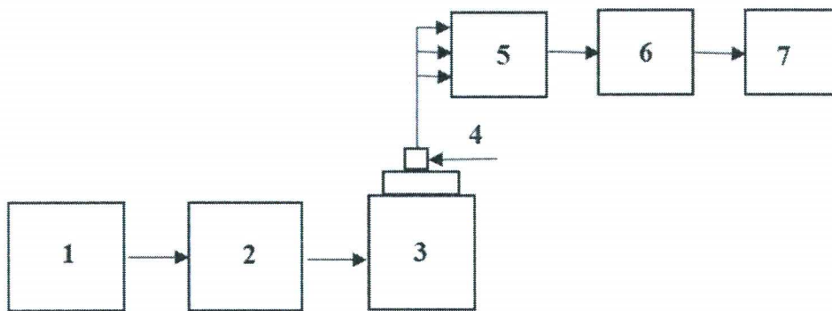
Рисунок 3 - Блок-схема виброустановки при определении относительного коэффициента поперечного движения вибростола виброустановки
