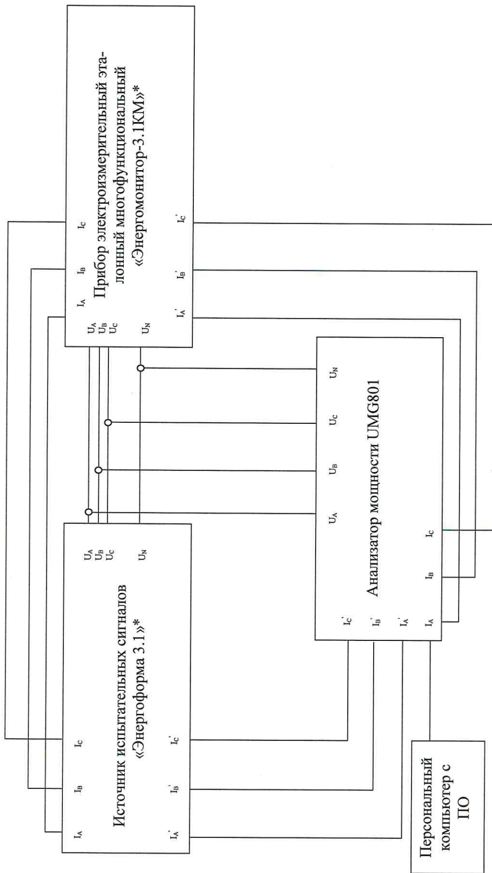
Рисунок 2 - Схема структурная определения метрологических характеристик
