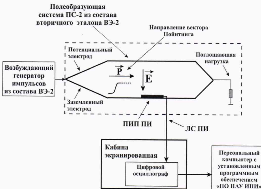
Рисунок 8 – Схема исследований при определении характеристик измерительных преобразователей с использованием вторичного эталона единиц напряженности импульсных электрического и магнитного полей ВЭ-2
