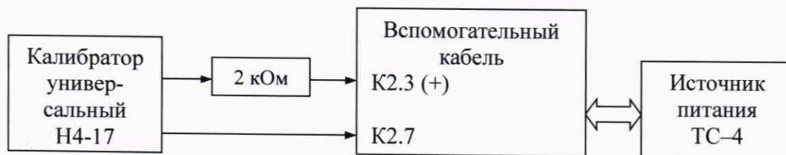
Рисунок 6 - Структурная схема соединения приборов
