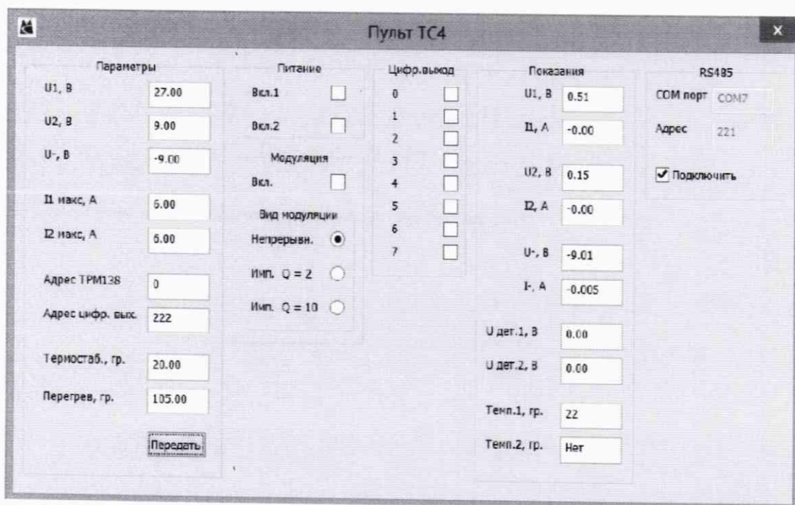
Рисунок 3 - Диалоговое окно программы «TS4Pult.exe»
