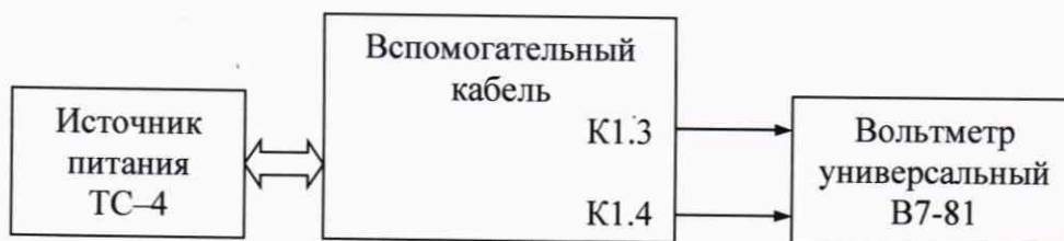
Рисунок 1 - Структурная схема соединения приборов
