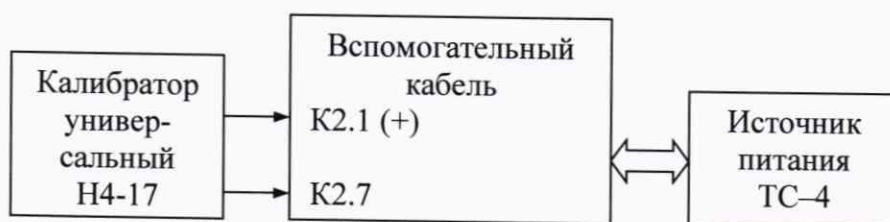
Рисунок 5 - Структурная схема соединения приборов
