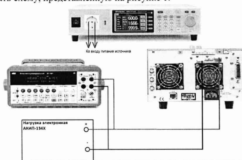
Рисунок 1 – Схема соединения приборов для определения метрологических характеристик источников питания в режиме стабилизации напряжения.
