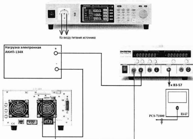
Рисунок 3 – Схема соединения приборов для определения метрологических характеристик источников питания в режиме стабилизации силы тока.
