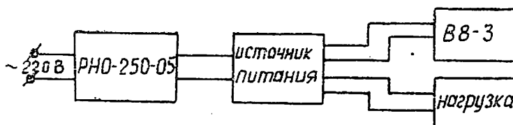
Рис. 4. Структурная схема измерения нестабильности выходного напряжения
