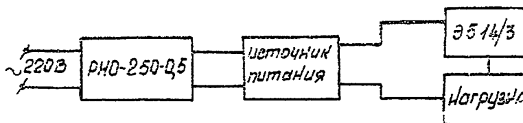
Рис. 6. Структурная схема измерения тока срабатывания защиты прибора
