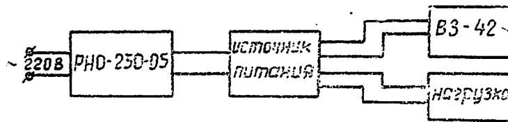
Рис. 5. Структурная схема измерения пульсации выходного напряжения
