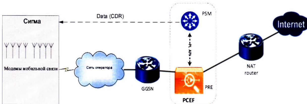
Рисунок 1 - Схема поверки СИПД
