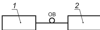
1 — проверяемый ОР; 2 — оптический генератор рабочего эталона (ОГ РЭ); ОВ — оптическое волокно
