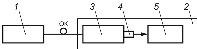
1 — проверяемый ОР; 2 — спектральная установка РЭСМ-ВС (СУ); 3 — монохроматор; 4 — фотоприемное устройство; 5 — регистратор, ОК — оптический кабель
