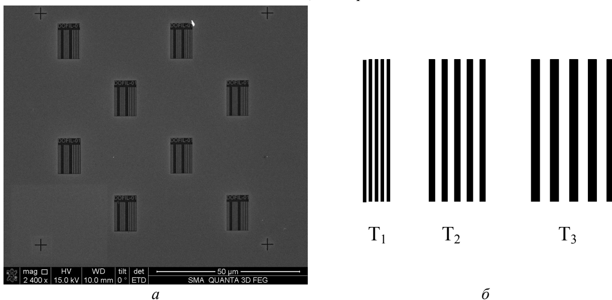
Рис.1 а – изображение электронно-микроскопическое рабочей области СО структуры нанопериодической DOFIL–01, представляющей собой расположенные в шахматном порядке ансамбли, упорядоченных наборов линий, длиной приблизительно 10 мкм и периодами T_1 , T_2 , T_3 , б – схематическое изображение одного из ансамблей с указанием периодов структуры: T_1 , T_2 , T_3 .
