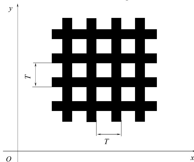
Рис.1 Схематическое изображение фрагмента поверхности СО структуры нанопериодической VSDU-500, представляющей собой ансамбль упорядоченно расположенных квадратных ямок, расположенных трансляционно-симметрично. Показана аттестуемая характеристика: период структуры T (без различия направлений Ox и Oy ).
