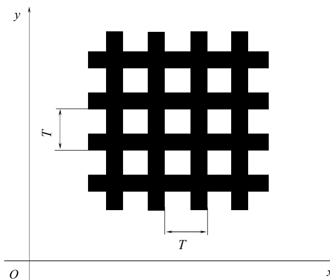
Рис.1 Схематическое изображение фрагмента поверхности СО структуры нанопериодической VSDU-1000, представляющей собой ансамбль упорядоченно расположенных квадратных ямок, расположенных трансляционно-симметрично. Показана аттестуемая характеристика: период T (без различения направлений Ox и Oy ).
