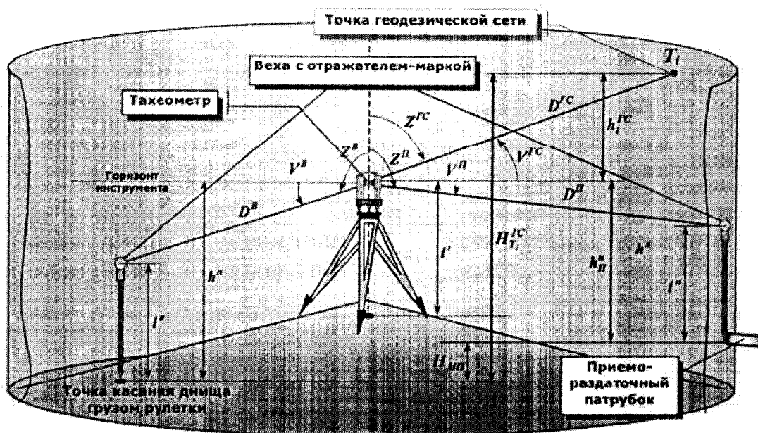
Рисунок А.3 Определение абсолютной высоты точки геодезической сети и „мертвой” полости относительно точки касания днища грузом рулетки при установке тахеометра внутри резервуара
