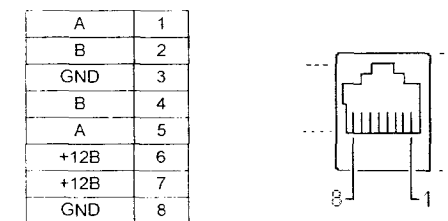
Рисунок А.3 Розетка питания и интерфейса RS-485
