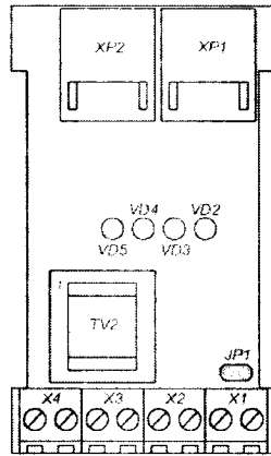
Рисунок 1.7 Плата клеммников модуля М-315
