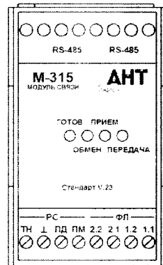
Рисунок 1.8 Модуль М-315
