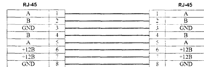
Рисунок А.1 Схема кабеля межмодульного соединения
