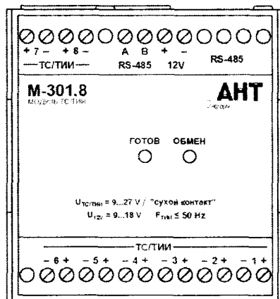
Рисунок 1.2 Модуль М-301.8
