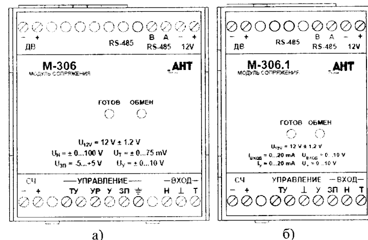
Рисунок 1.10. Модули М-306 (а) и М-306.1 (б)
