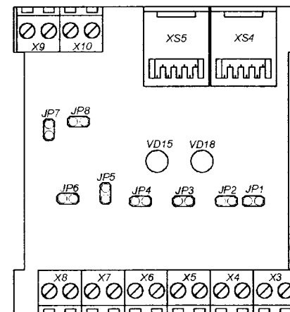
Рисунок 1.4 Плата клеммников модуля М-302.8
