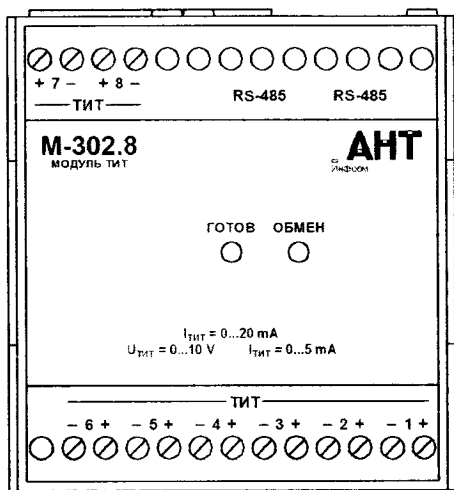
Рисунок 1.5 Модуль M-302.8
