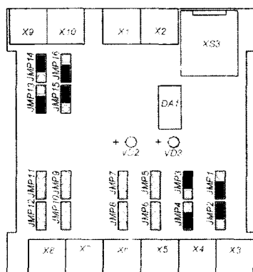
Рисунок 1.3 Плата клеммников модуля М-301.8
