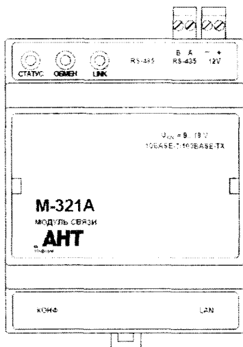
Рисунок 1.9 Внешний вид модуля M-321A
