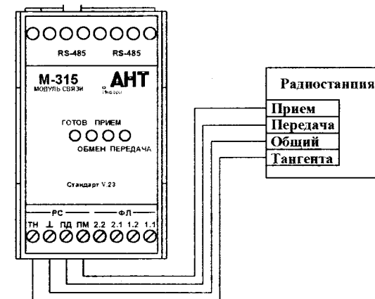
Рисунок 2.1 Подключение радиостанции
