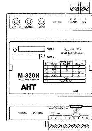
Рисунок 1.1 Модуль М-320И
