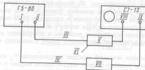
Рис. 41. Схема соединения приборов при измерении длительности фронта и среза импульсов:
