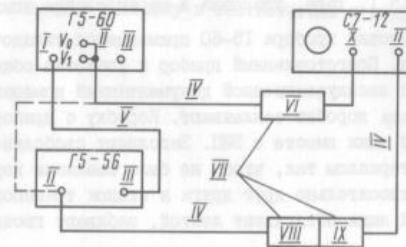
Рис. 42. Схема соединения приборов для определения параметров синхроимпульсов V_0 и V_I : I — внешний запуск; II — синхронизация; III — выход; IV — кабель В4 № 2; V — кабель В4 № 4; У1 — аттенуатор 10 дБ; У3 — из комплекта осциллографа С7-12; У3 — аттенуатор 20 дБ; IX — переход Э2-И2/2; X — вход
