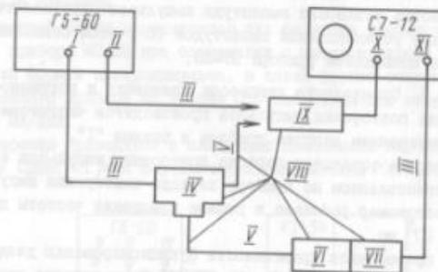
Рис. 39. Схема соединений приборов при измерении длительности импульсов в режиме "3":
