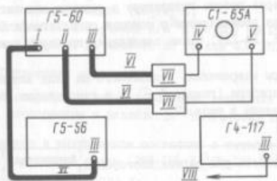
Рис. 37. Схема соединения приборов при проверке режима внешнего запуска:
