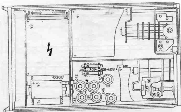
Рис. 3. Схема расположения установочных элементов и печатных плат (вид снизу)
