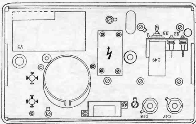
Рис. 5. Газная стрелка осциллографа. Расположение установочных элементов и печатных плат
