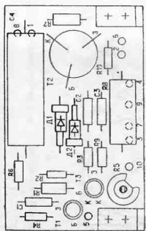
Рис. 10. Маркировочная схема платы высоковольтного преобразователя.
