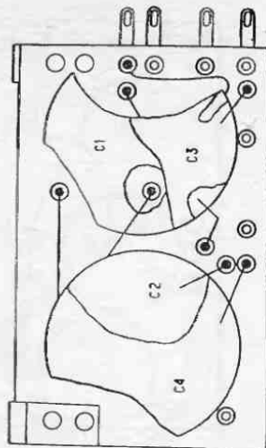
Рис. 14. Маркировочная схема выпрямителя высоковольтного 1,5 кВ.
