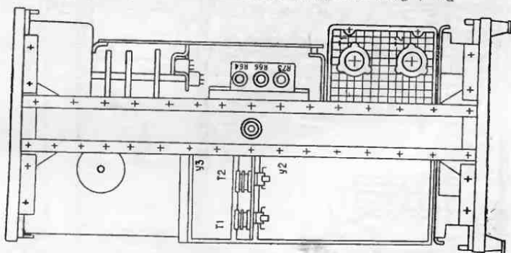
Рис. 4. Схема расположения установочных элементов (вид сверху)
