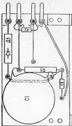
Рис. 11. Маркировочная схема высоковольтного усилителя.
