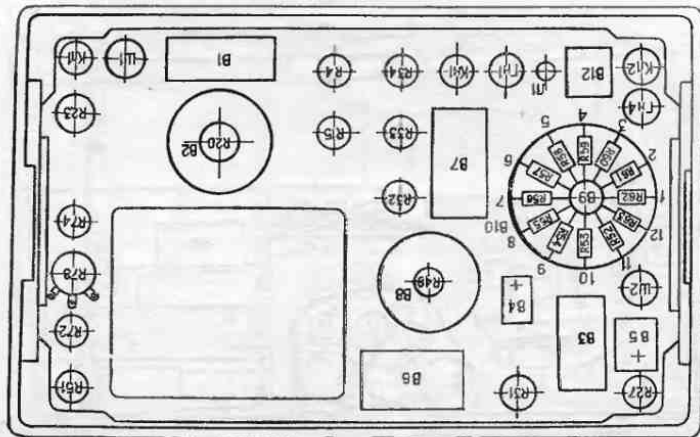
Рис. 1. Передняя панель осциллографа (мд сэлм). Схема расположения установочных элементов
