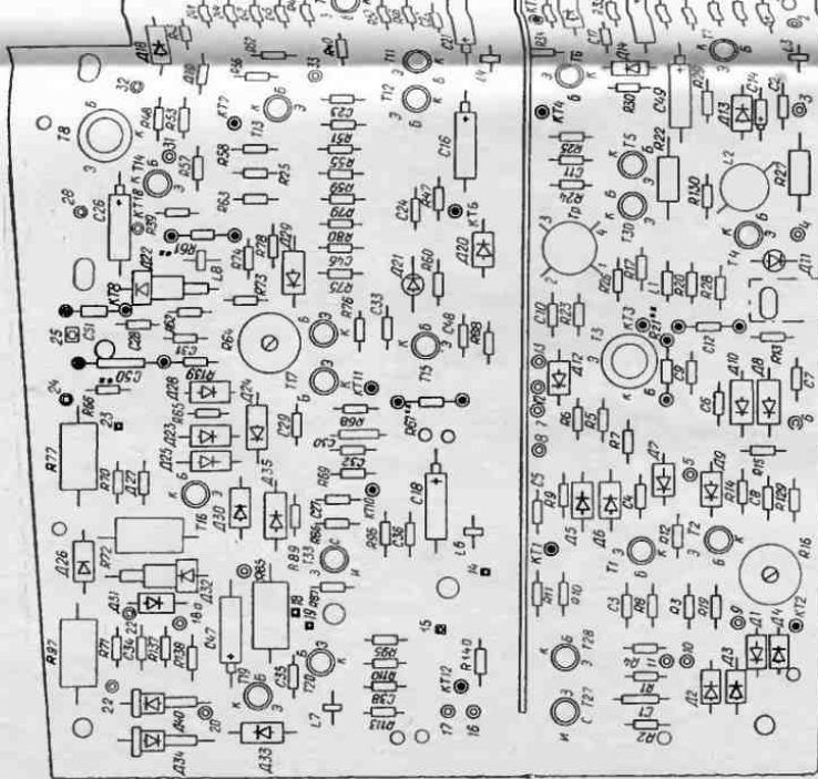
Рис. 5. Маркировочная схема блока развертки, делителя и усилителя горизонтального отклонения.
