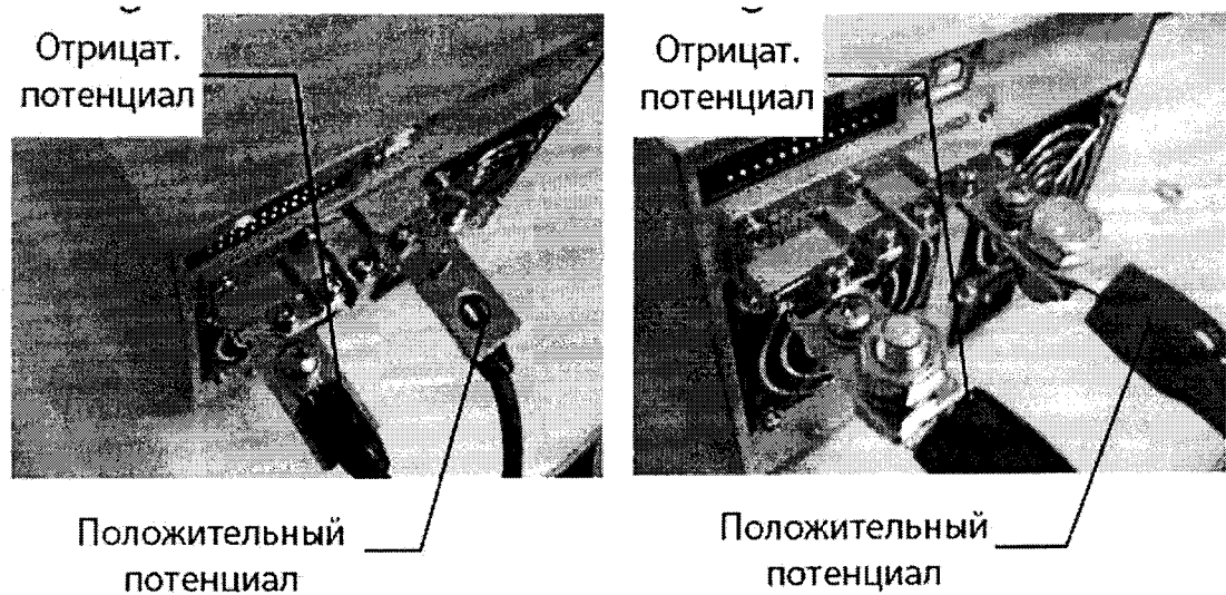
Рисунок 1 – Соединения проводов с клеммами источника
