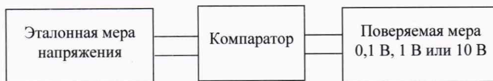
Рисунок 1 – Схема сличения поверяемой меры с эталонным СИ
