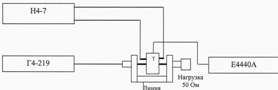
Рисунок 6 – Схема подключения
