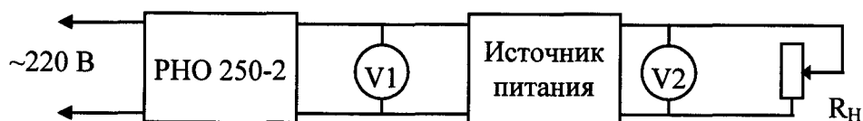
Рис. 3. Структурная схема определения пульсации выходного напряжения в режиме стабилизации напряжения.
