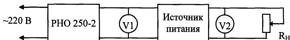
Рис. 1. Структурная схема определения основной погрешности измерения выходного напряжения.
