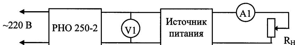
Рис. 4а. Структурная схема определения основной погрешности измерения выходного тока до 3 А.
