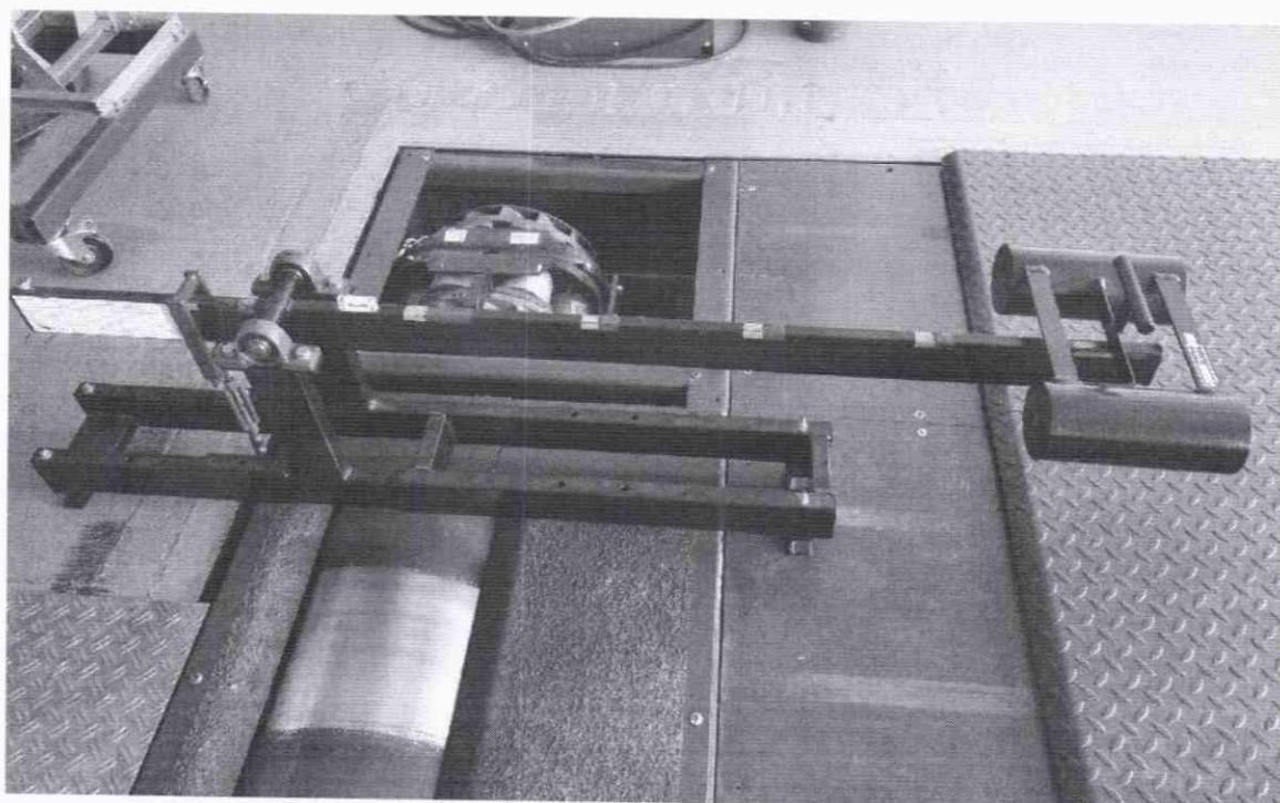
Рисунок 4 - Схема установки калибровочного рычага для модификации MSR 500 и MSR 400. (А - калибровочный вес; В - калибровочный рычаг; С - пузырьковый уровень; D - резьбовая тяга; Е - гибкая тяга; F – винт)
