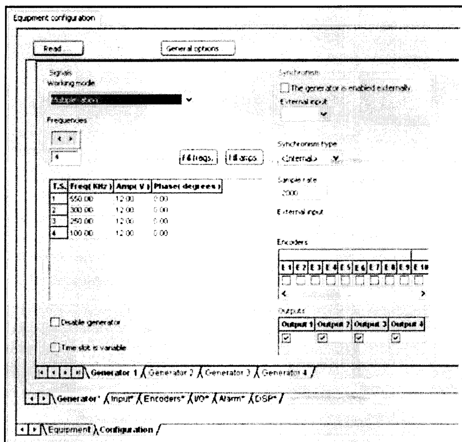
Рисунок 2 - Конфигурация генератора в дефектоскопе
