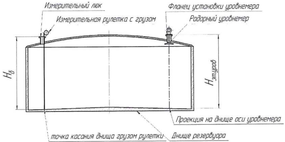
Рисунок А.1 – Схема измерения базовой высоты резервуара РВС-5000 и эталонного расстояния уровнера
