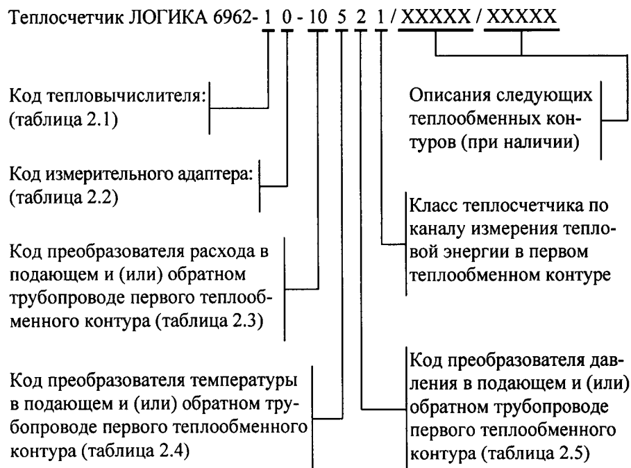
Рисунок 2.1 – Структура обозначения исполнений теплосчетчиков
