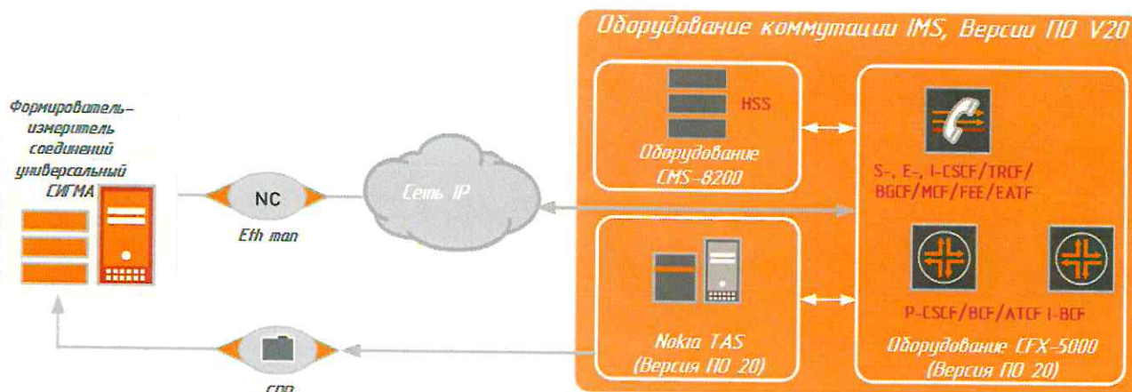
Рисунок 1- Схема поверки
