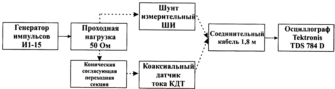
Рисунок 1 – Схема определения метрологических характеристик шунта измерительного ШИ и коаксиального датчика тока КДТ
