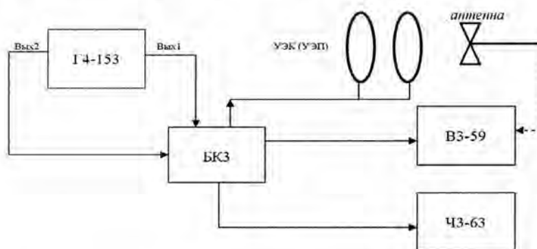
Рисунок 1 - Структурная схема измерений коэффициента калибровки электрической антенны в диапазоне частот от 9 кГц до 30 МГц
