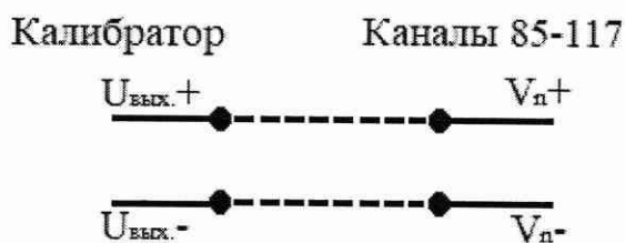
Рисунок 7 – Схема подключения калибратора к каналам измерения аналогового ввода для измерения напряжения.
