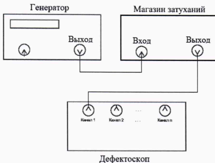
Рисунок 28 – Схема подключения.
