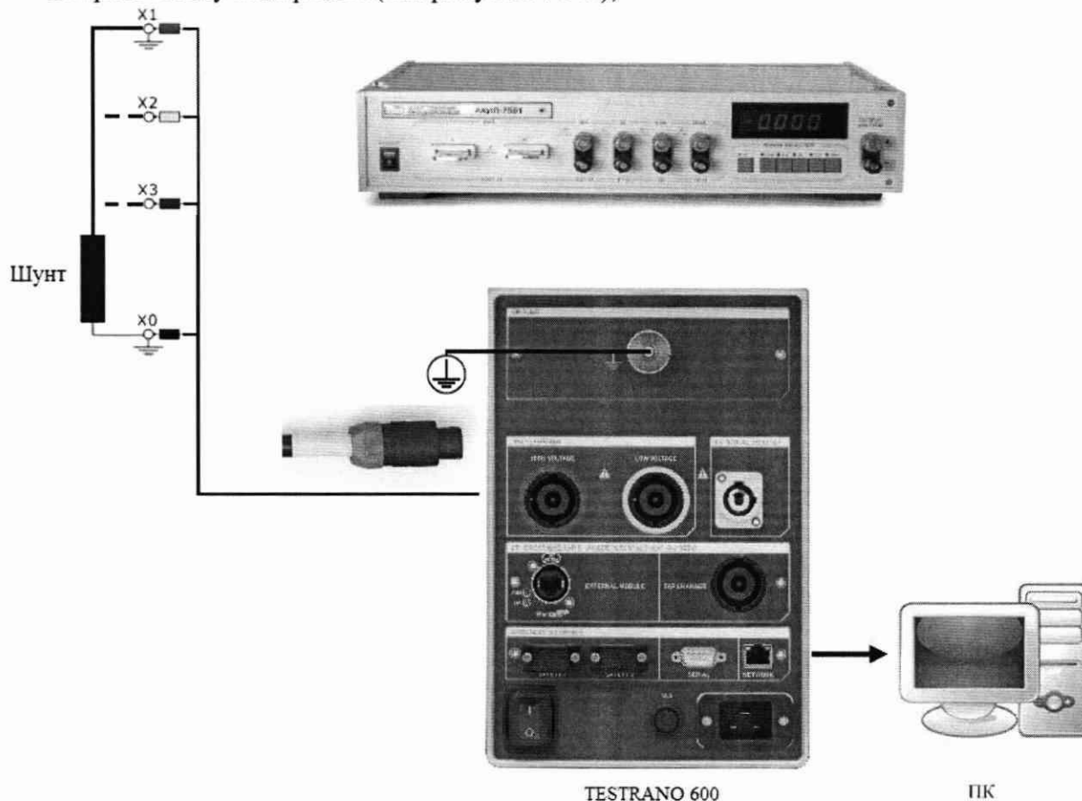
Рисунок 7.9.1 – Структурная схема соединения приборов для определения абсолютной погрешности измерений сопротивления постоянному току (конфигурируемый выход «LOW VOLTAGE»)
