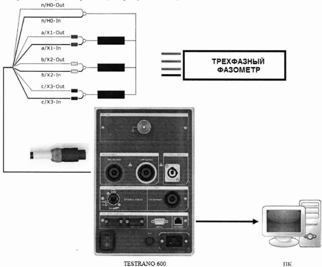
Рисунок 7.8.1 – Структурная схема соединения приборов для определения пределов допускаемой абсолютной погрешности воспроизведения / измерений фазового угла источниками / входами тока (конфигурируемый выход «LOW VOLTAGE»)
