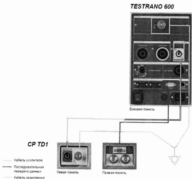
Рисунок 7.10.1 – Структурная схема соединения CP TD1 (CP TD12, CP TD15) и TESTRANO 600 для определения абсолютной погрешности измерений электрической емкости и тангенса угла диэлектрических потерь
