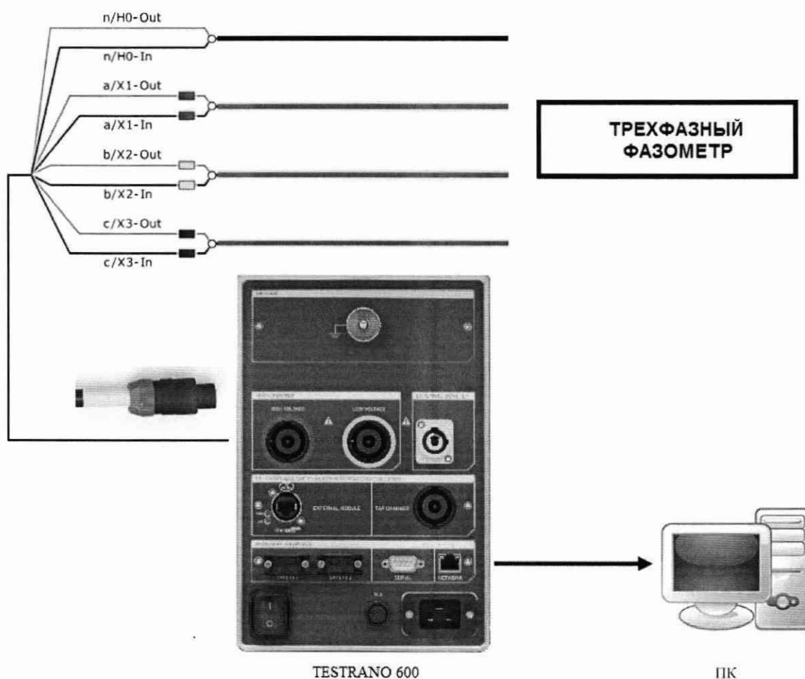
Рисунок 7.8.3 – Структурная схема соединения приборов для определения пределов допускаемой абсолютной погрешности воспроизведения / измерений фазового угла источниками / входами напряжения (конфигурируемый выход «LOW VOLTAGE»)
