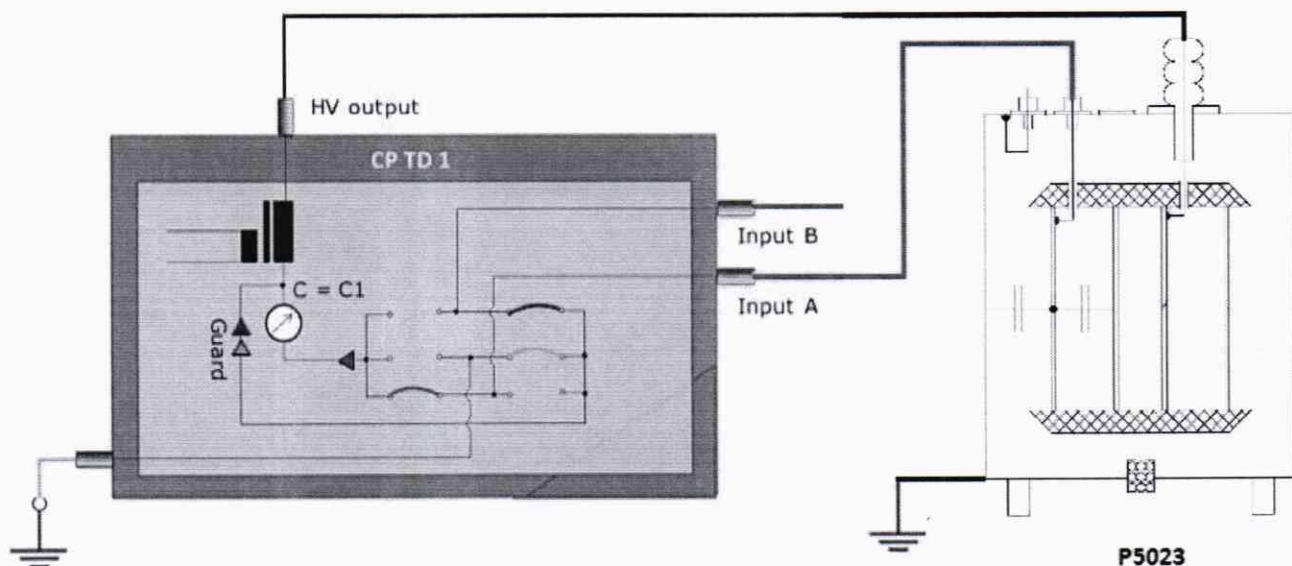
Рисунок 7.10.2 – Структурная схема соединения приборов для определения абсолютной погрешности измерений электрической емкости и тангенса угла диэлектрических потерь
