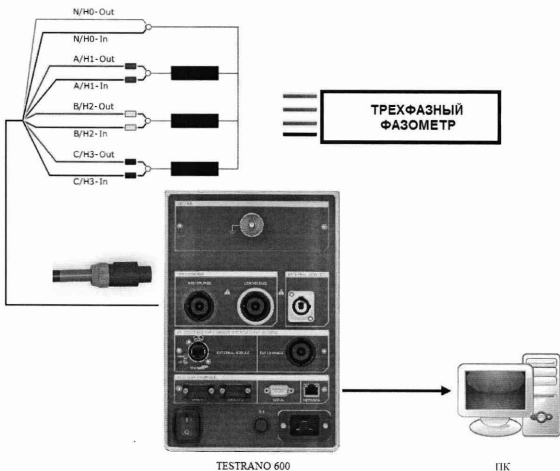
Рисунок 7.8.2 – Структурная схема соединения приборов для определения пределов допустимой абсолютной погрешности воспроизведения / измерений фазового угла источниками / входами тока (конфигурируемый выход «HIGH VOLTAGE»)
