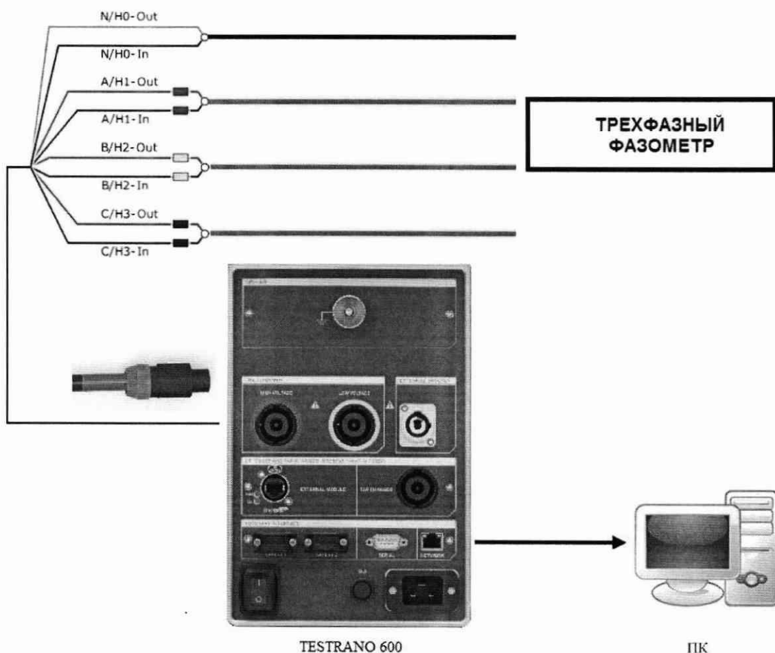
Рисунок 7.8.4 – Структурная схема соединения приборов для определения пределов допустимой абсолютной погрешности воспроизведения / измерений фазового угла источниками / входами напряжения (конфигурируемый выход «HIGH VOLTAGE»)
