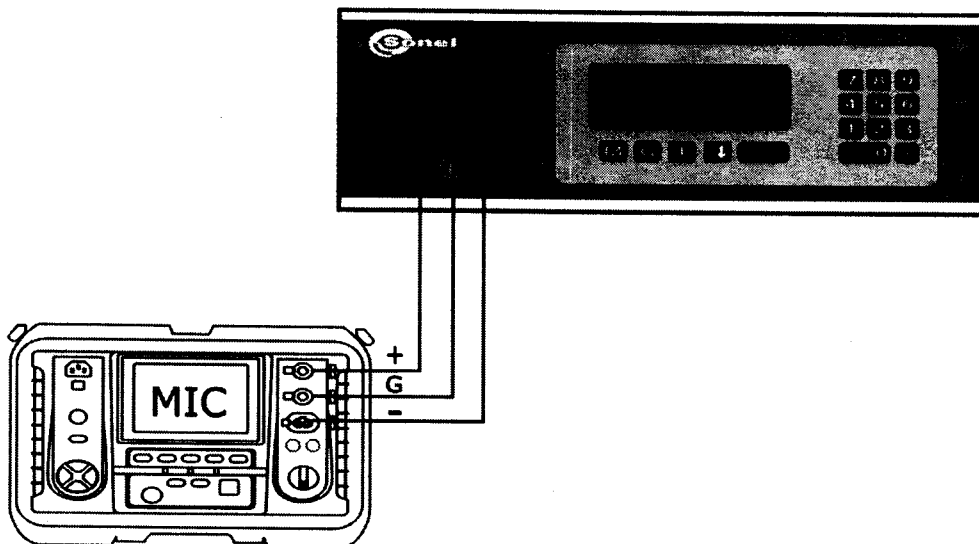
Рисунок 2 - Структурная схема определения абсолютной погрешности измерения сопротивления электроизоляции до 5 ТОм
