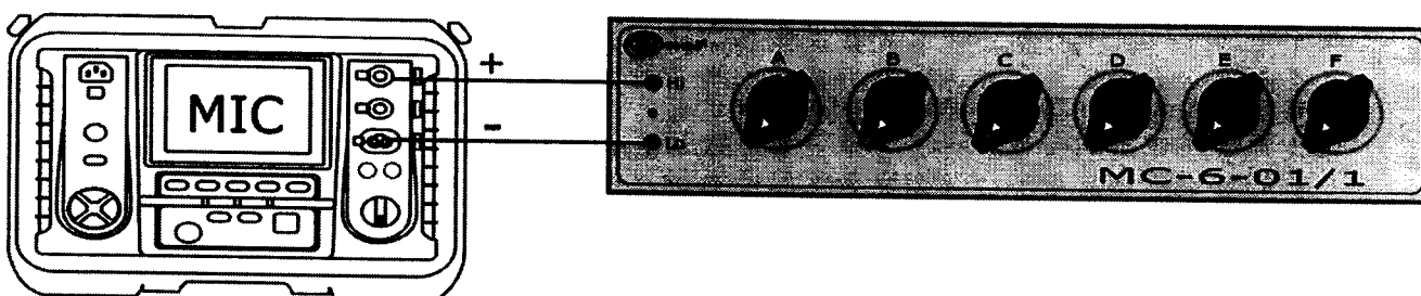
Рисунок 5 - Структурная схема определения абсолютной погрешности измерения сопротивления защитных проводников где MIC – поверяемый измеритель MIC-5010; MC-6-01/1 – магазин электрического сопротивления MC-6-01/1.
