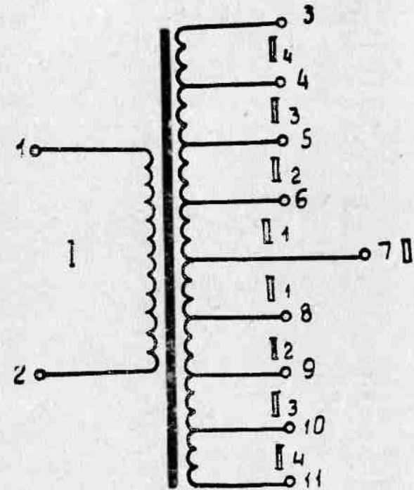
Рис. 2. Схема электрическая принципиальная трансформатора согласующего низкочастотного тороидального
