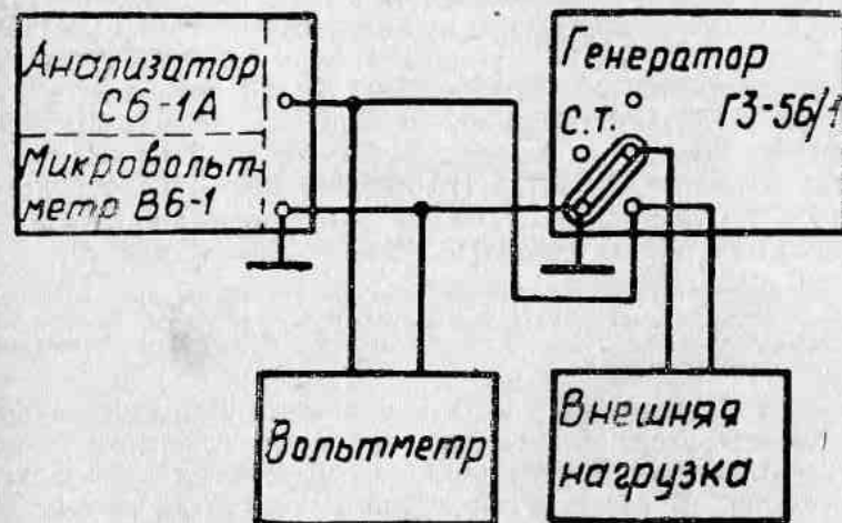
Рис. 7. Схема электрическая структурная проверки K_r на внешних нагрузках
