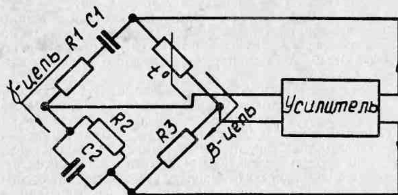
Рис. 2. Схема электрическая структурная задающего генератора.
