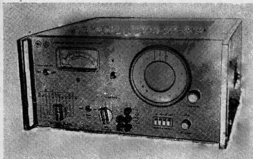
Общий вид генератора ГЗ-56/1
