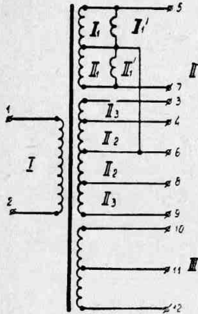
Рис. 1. Схема электрическая принципиальная трансформатора согласующего высокочастотного тороидального
