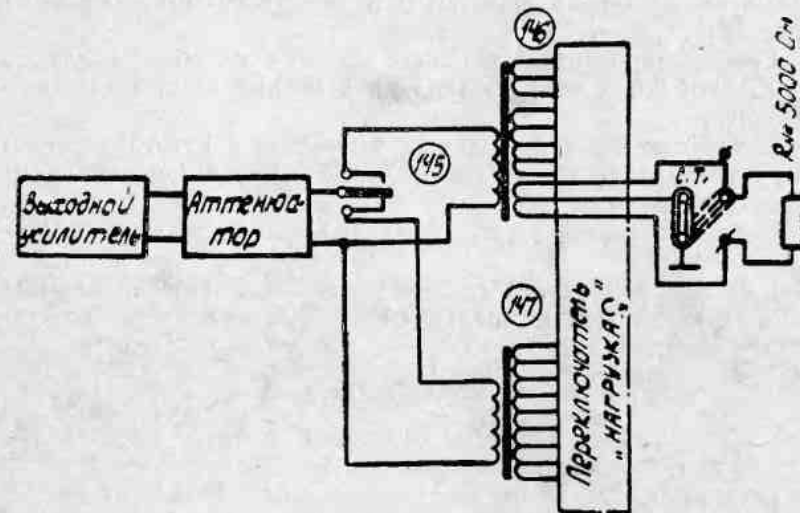
Рис. 3. Схема структурная электрическая дополнительного выхода генератора
