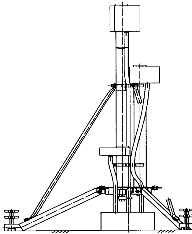
Рисунок 1.1 - Установка периодической поверки ФТЕИ.407619.003
