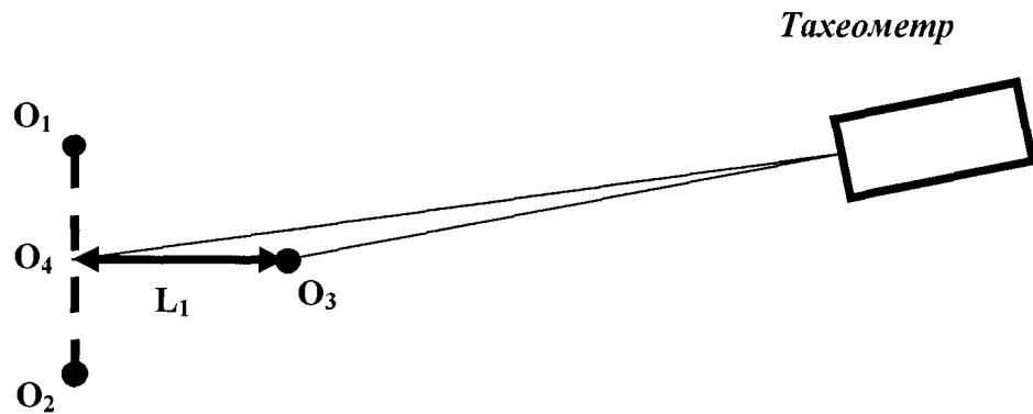
Рисунок 3 - Схема измерений (угол крена)
