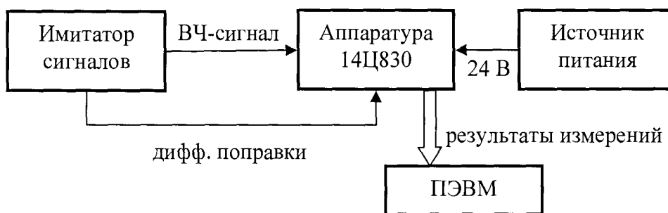
Рисунок 1 Схема измерений
