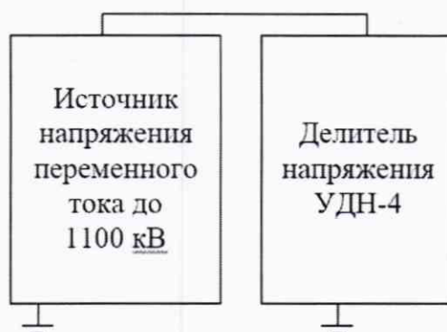
Рисунок 1 – Схема проверки электрической прочности
