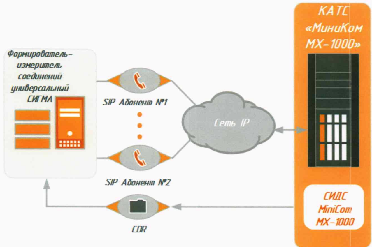
Рисунок 1- Схема поверки
