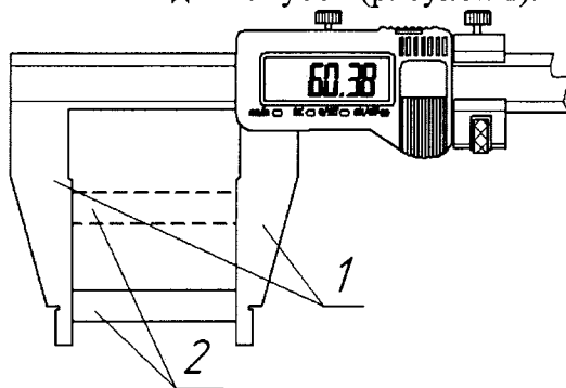
1 – губки штангенциркуля; 2 – концевая мера длины
