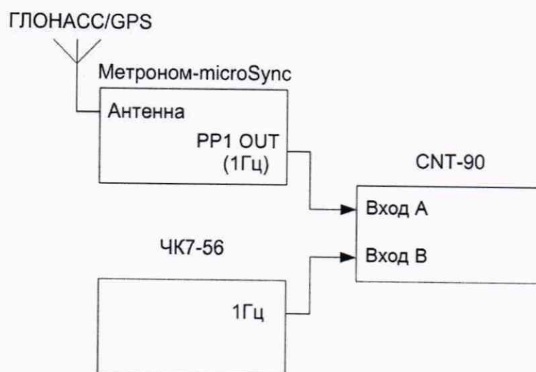
Рисунок 2 – Схема для измерения абсолютной погрешности формирования шкалы времени относительно шкалы времени UTC (SU)
