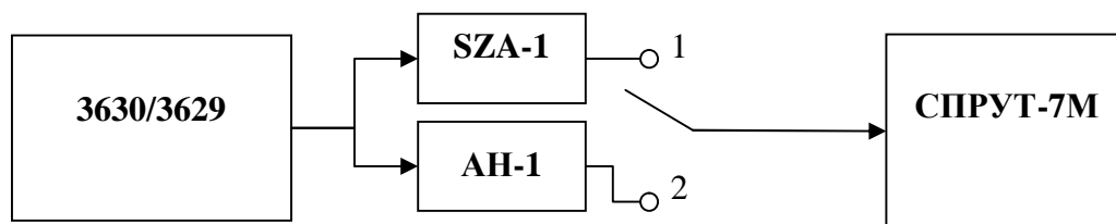
Рисунок 3 – Схема подключения
