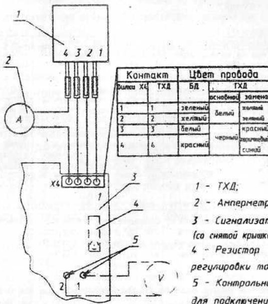
Рисунок 11.2 - Схема подключения амперметра к ТХД для установки рабочего тока
