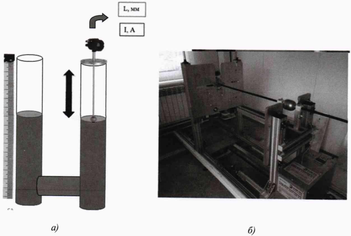
Рисунок 1 – Проверка преобразователя на поверочной установке а) с непосредственным изменением уровня жидкости б) с имитацией изменения уровня жидкости
