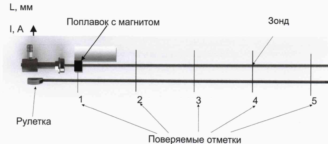
Рисунок 3 – Проверка преобразователя с помощью рулетки и магнитного поплавка
