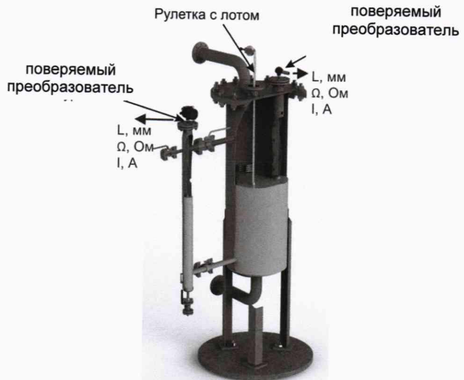
Рисунок 2 – Проверка преобразователя без демонтажа с помощью эталонной рулетки с лотом
